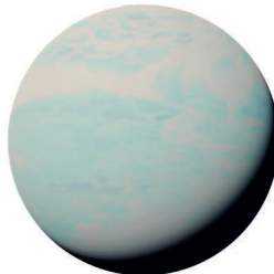
Der Uranus
