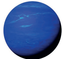
Der Neptun
