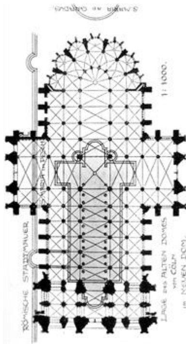
M3 - Kölner Dom, Grundriss und Spitzbogen (commons.wikimedia.org)
