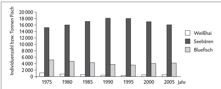
Abb. 1: Populationsentwicklung des Weißhais, des südafrikanischen Seebären und des Bluefish in der Region Natal, einer Provinz in Südafrika (beim Weißhai und Seebär handelt es sich um geschätzte reale Zahlen der vorkommenden Tiere, beim Bluefish sind die Fangergebnisse in Tonnen angegeben)
